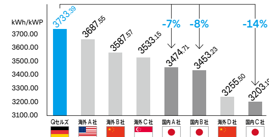
1kWあたり実発電量合計の比較 (一部抜粋)
